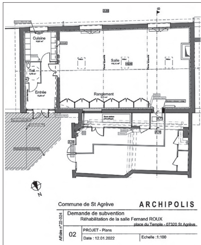
Plan projet de la salle Fernand Roux
